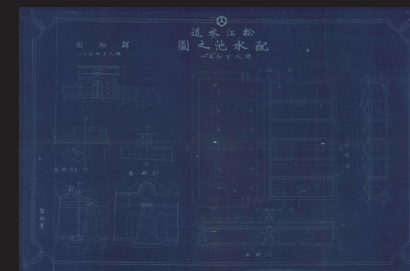
12. 配水池之圖
