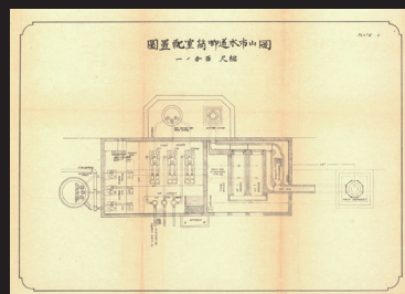
10. 岡山市水道唧筒室配置圖
