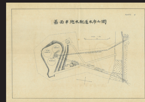
17. 岡山市水道配水池平面圖
