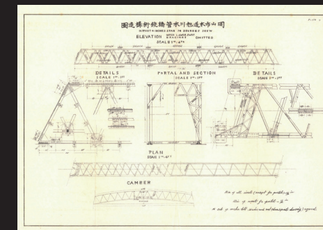
21. 岡山市水道旭川水管橋鉄桁構造圖
