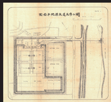
7. 岡山市水道水源地平面圖
