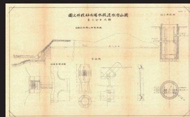
6. 岡山市水道取水場及砂取井之圖
