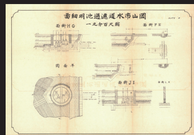
8. 岡山市水道濾過池明細圖
