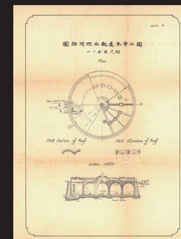
18. 岡山市水道配水池明細圖
