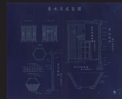
19. 量水室建築圖
