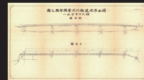
20. 岡山市水道旭川水管橋架橋之圖
