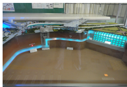
白子川地下調節池模型（東京都建設局所蔵）
